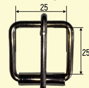
2489 Ø 3,5
